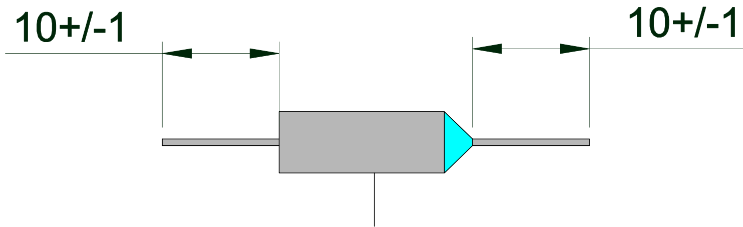
Bezpiecznik termiczny BF 157
