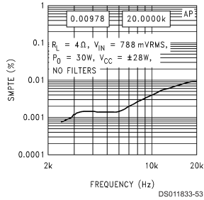
IMD 60 Hz, 1:1
